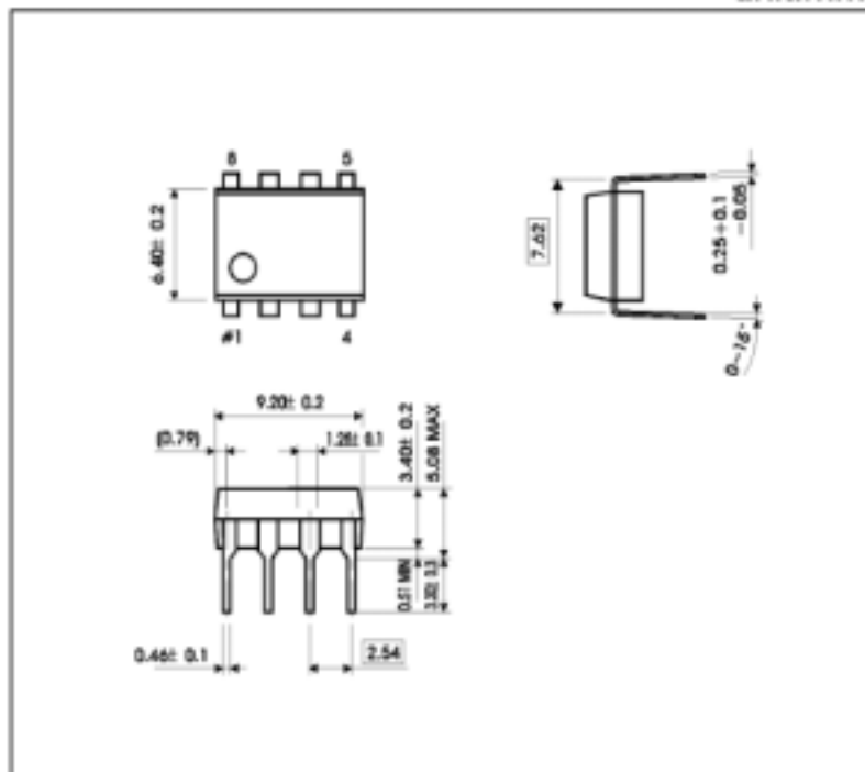
DIP-8
